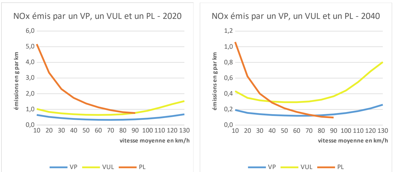
Illustration 8 : Comparaison des émissions de NOx en 2020 et en 2040 d'un VP, d'un VUL et d'un PL en fonction de la vitesse
